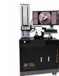
工具・砥石画像測定顕微鏡 TL-500H Plus
